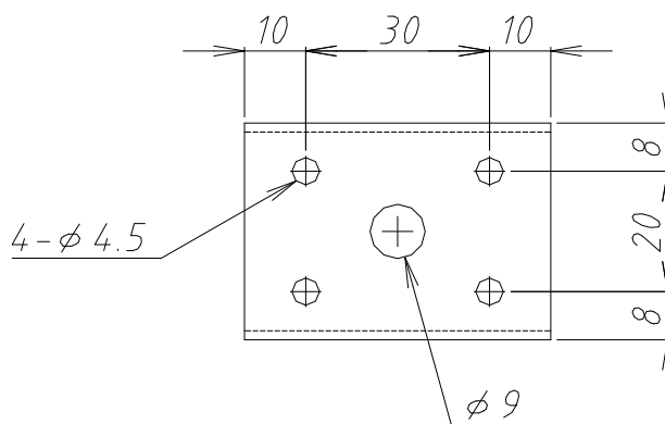
底面取付穴詳細図
